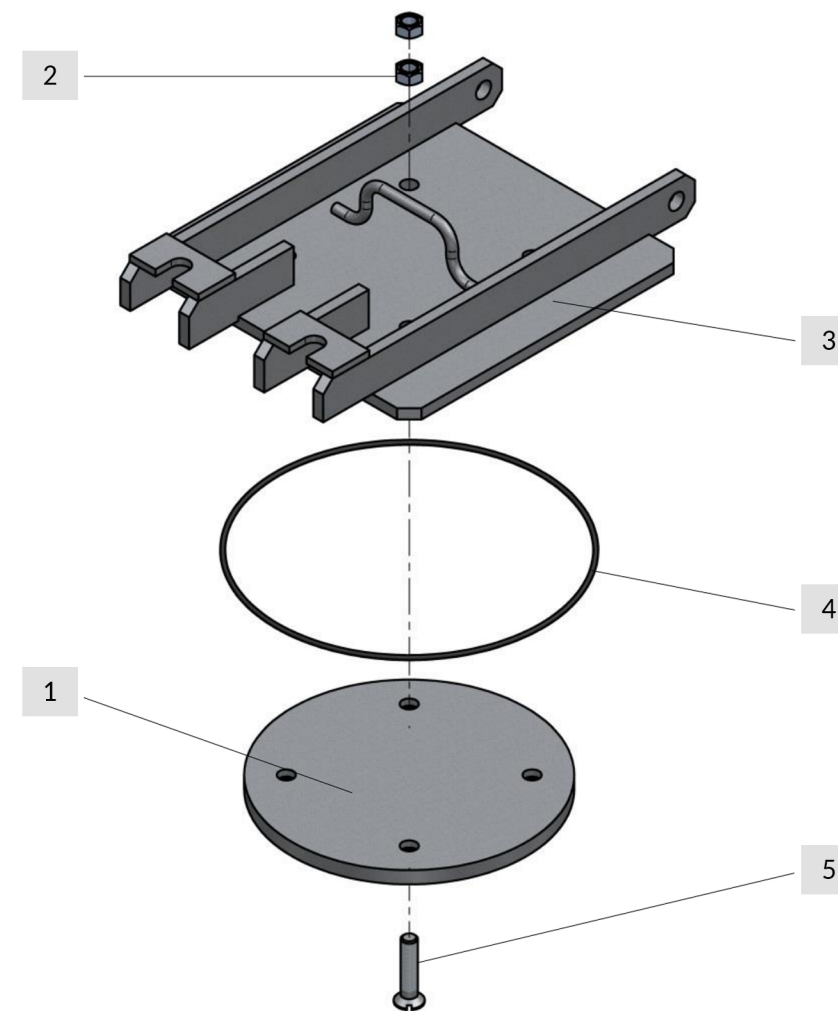
РИС. 5. ДСМД-75.02.11 – ДВЕРКА
