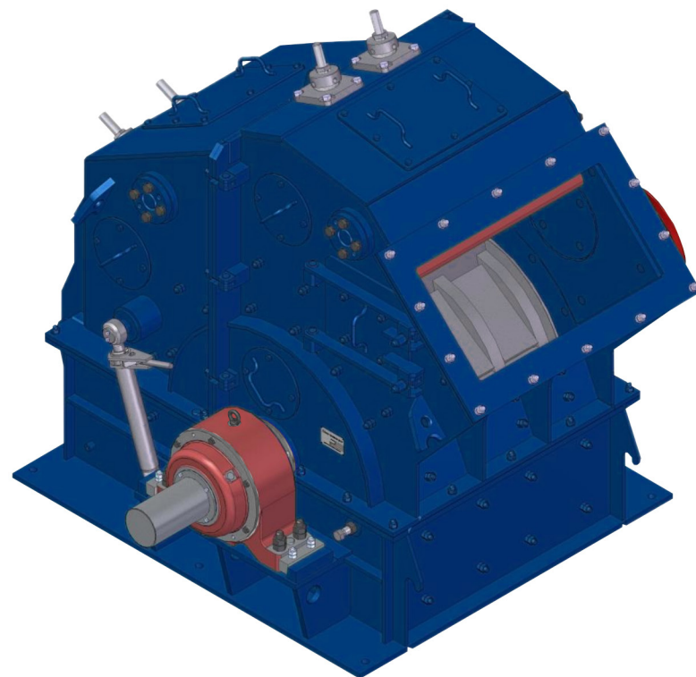
РИС. 1Б. ДСМД-75.01.01 – ДРОБИЛКА РОТОРНАЯ ДСМД-75 (ОБЩИЙ ВИД В СБОРЕ БЕЗ ЛОТКА)
